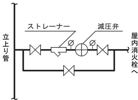
(減圧弁)
