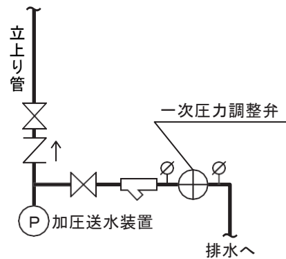
(一次圧力調整弁)
