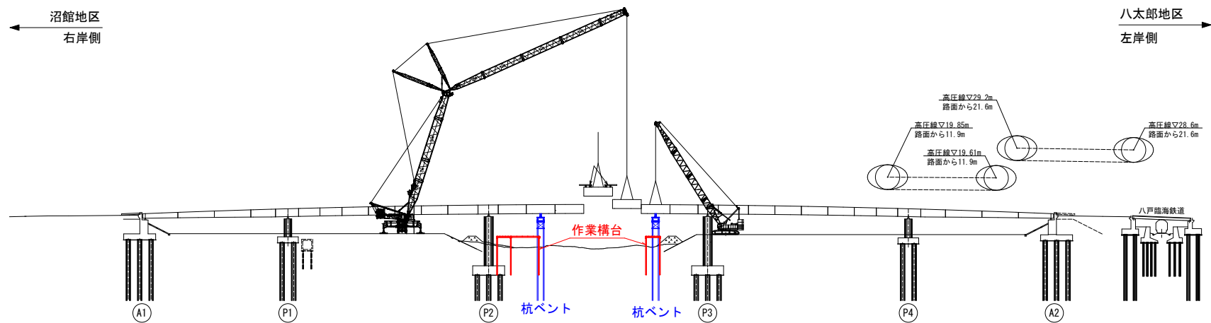
【側面図】
