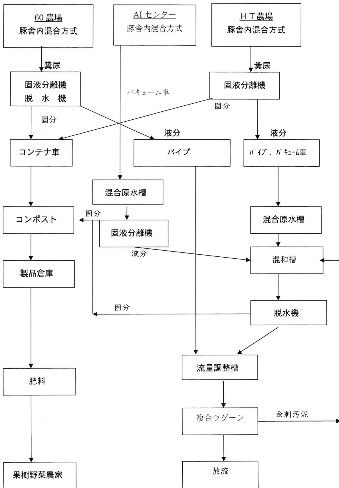
廃棄物処理フロー図
