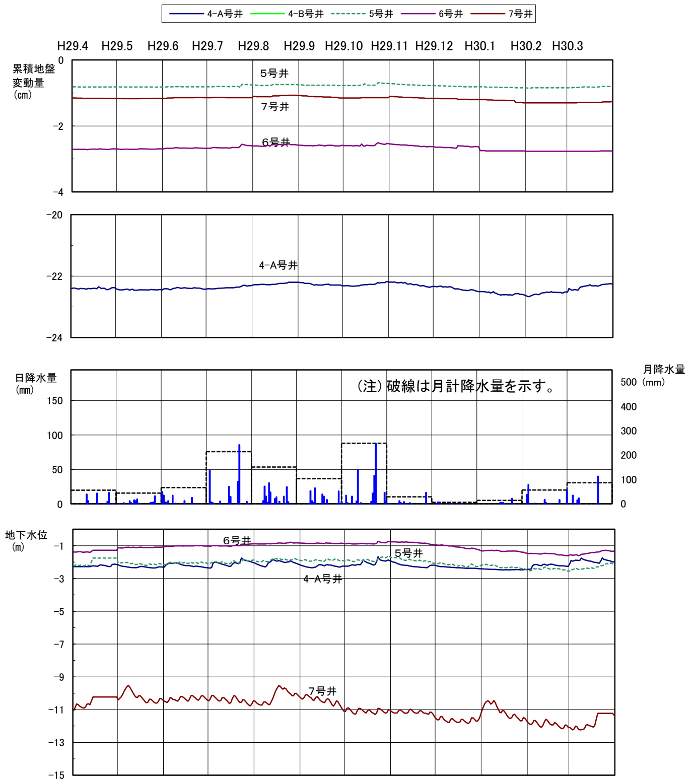
図5 平成29年度 累積地盤変動量と地下水位、降水量の関係
