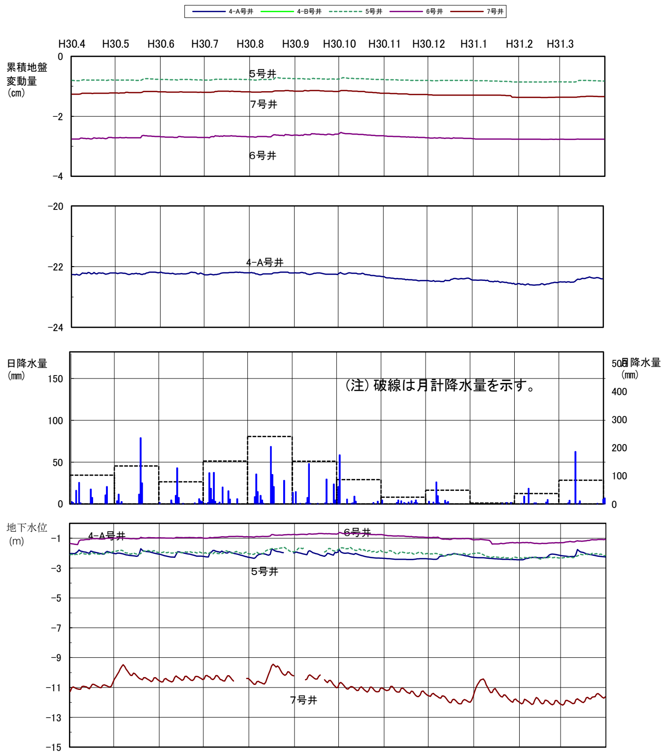
図6 平成30年度 累積地盤変動量と地下水位、降水量の関係
