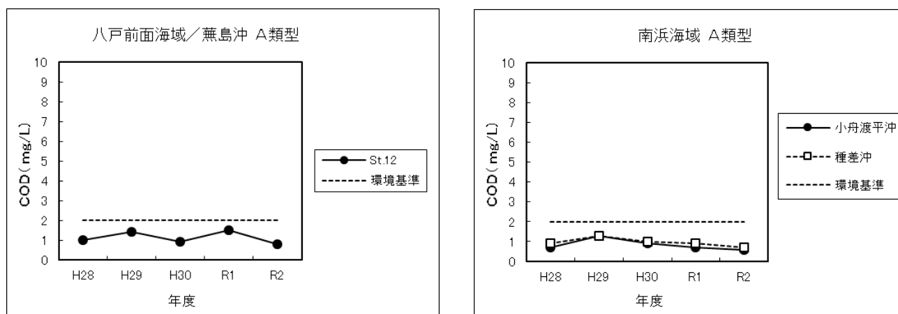
図1-4 海域のCOD経年変化
