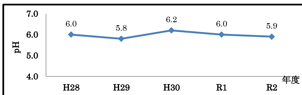
図 9 降雪の水素イオン濃度 (pH) 経年変化
