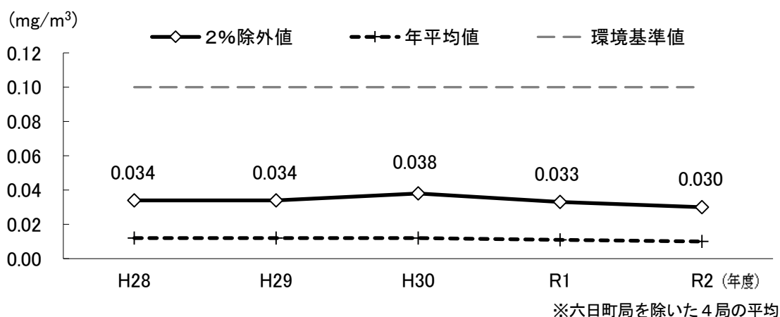
図2-4 浮遊粒子状物質の推移
