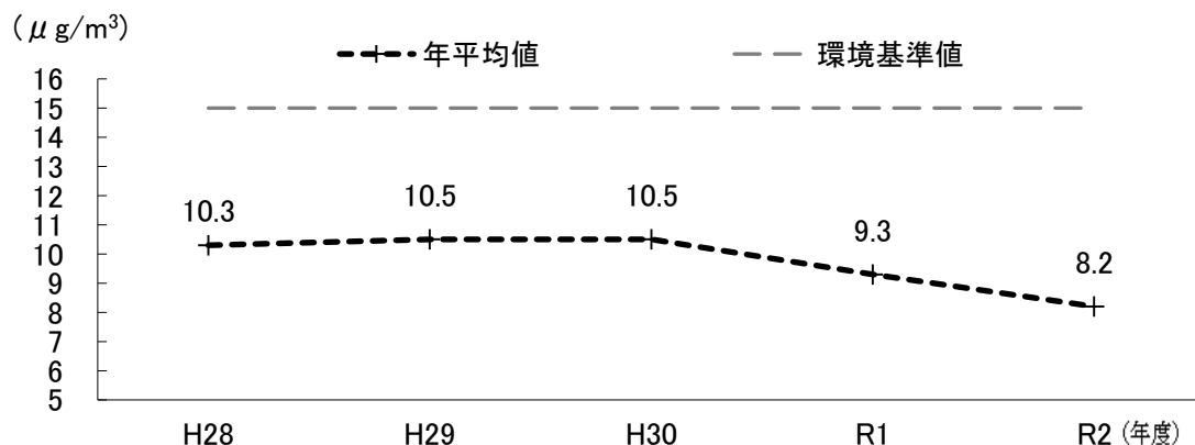
図 2-6 微小粒子状物質の推移
