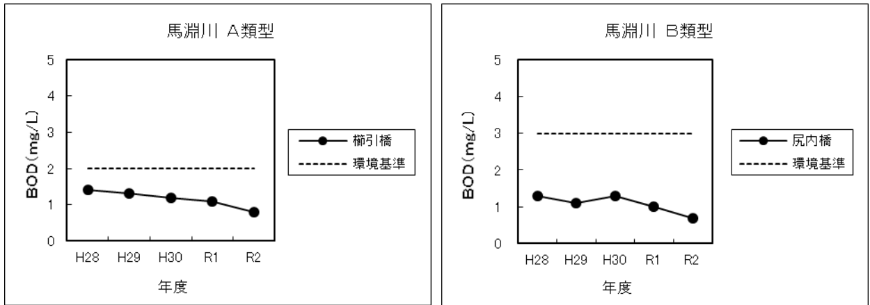
図1-2 馬淵川のBOD経年変化
