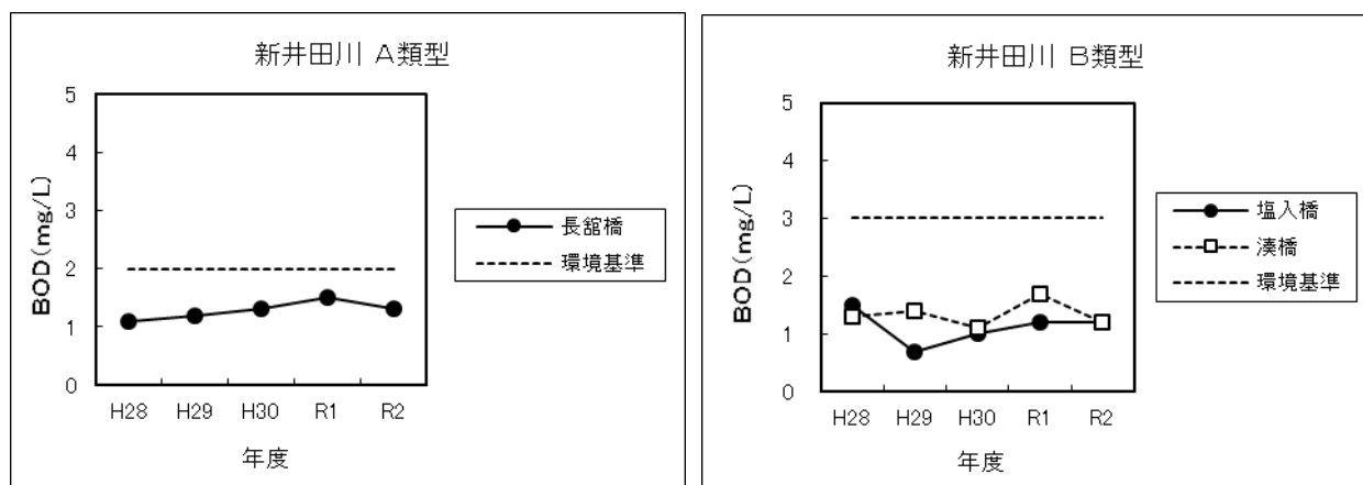
図1-1 新井田川のBOD経年変化
