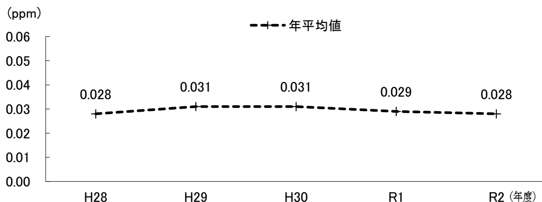
図 2-5 光化学オキシダントの推移
