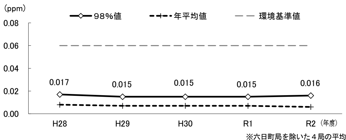
図2-3 二酸化窒素の推移
