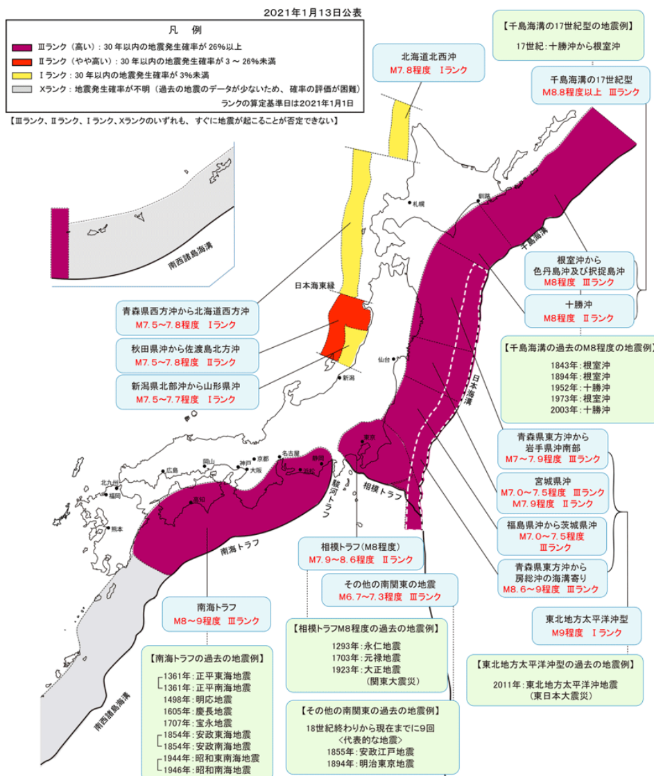
図56 主な海溝型地震の評価結果
