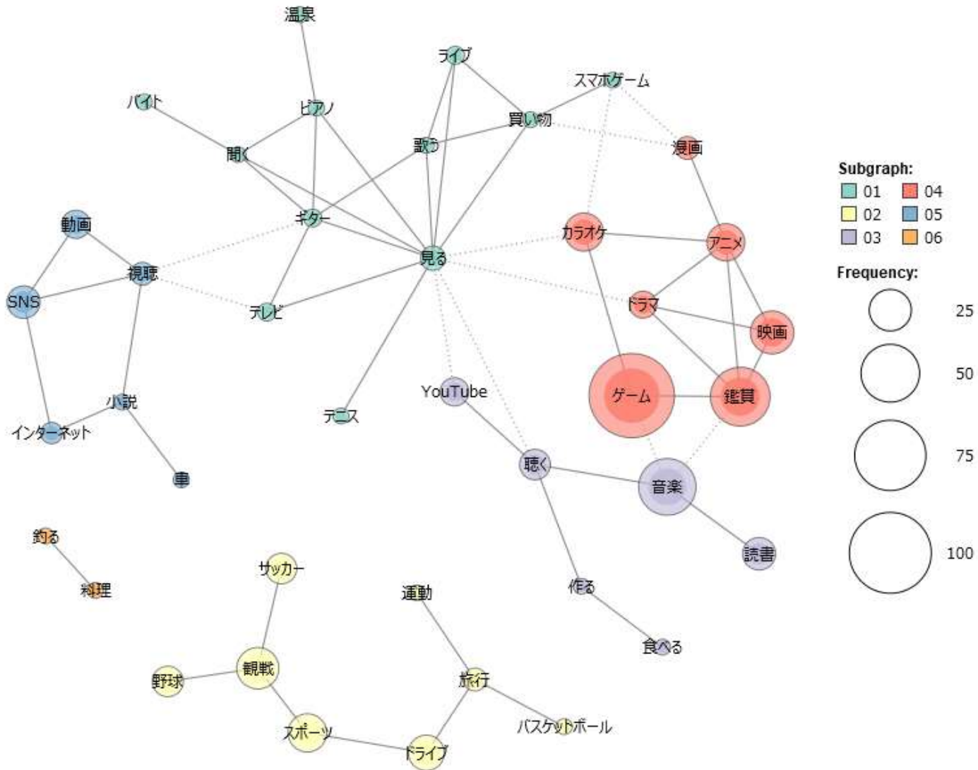
Q11サブグラフ(モジュラリティ)
