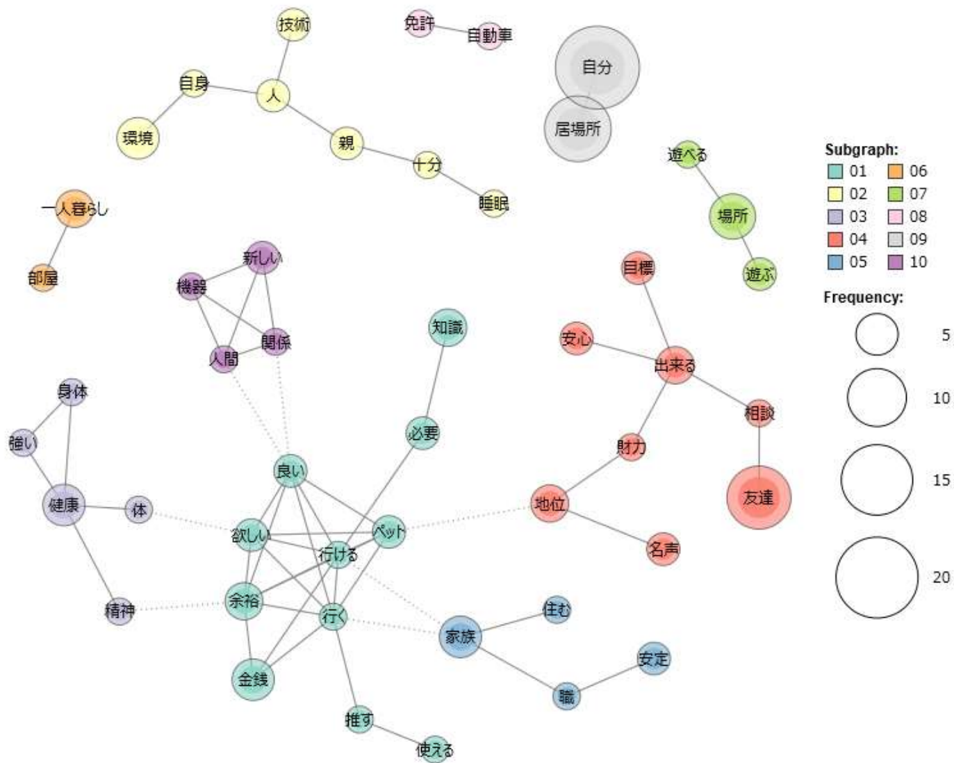
Q6サブグラフ(モジュラリティ)
