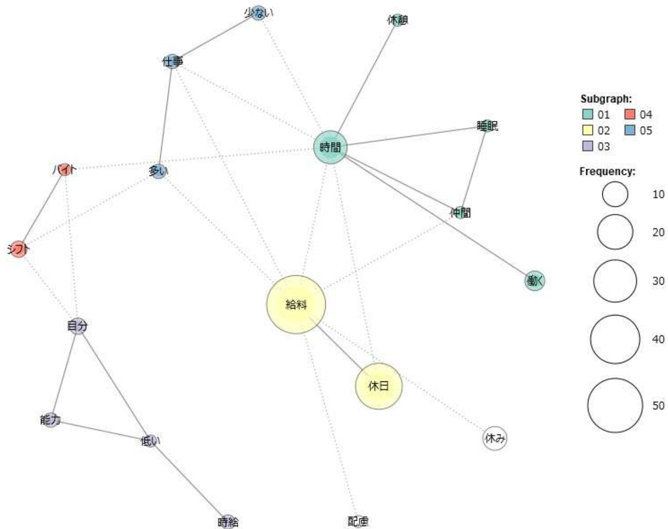
Q8サブグラフ(モジュラリティ)
