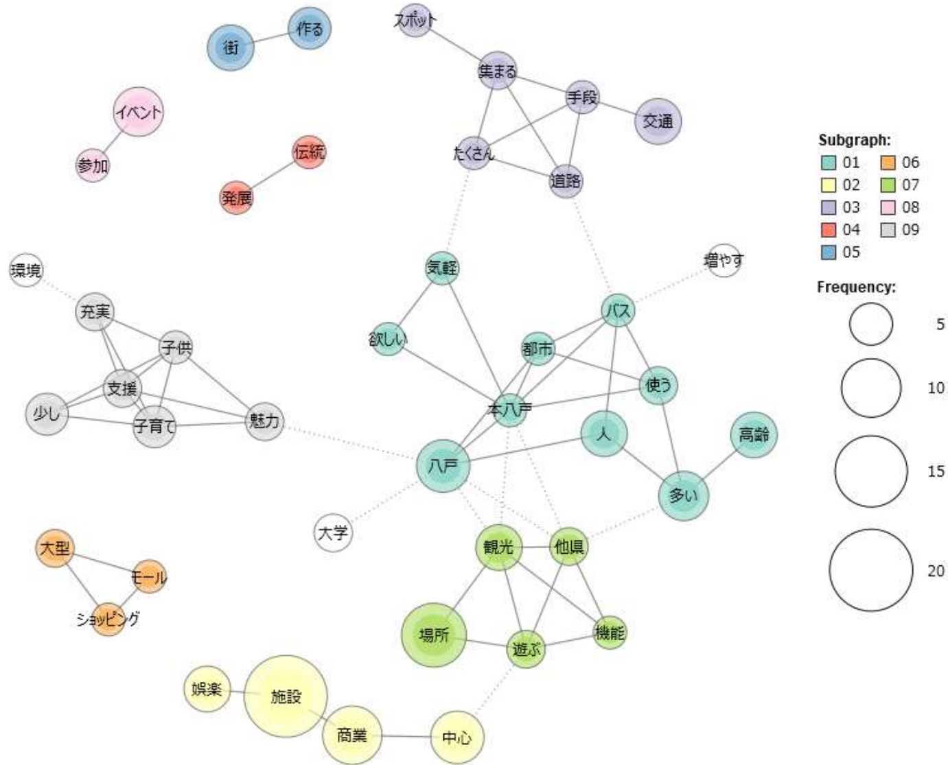
Q27サブグラフ(モジュラリティ)
