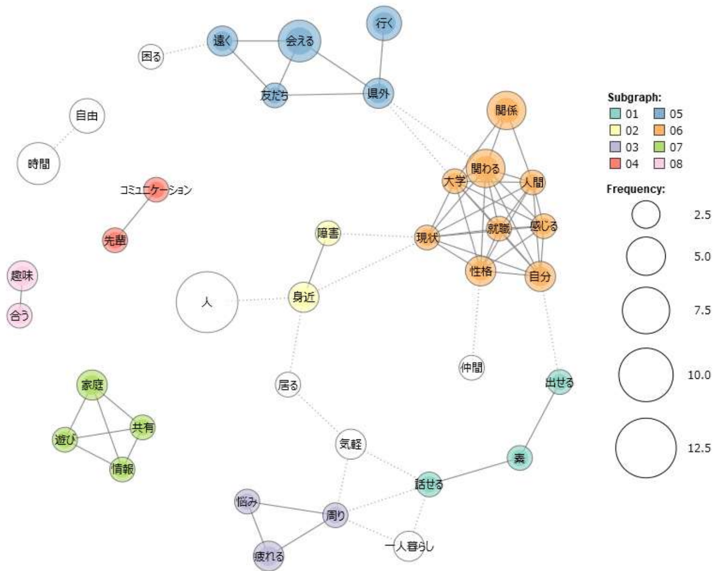
Q10サブグラフ(モジュラリティ)
