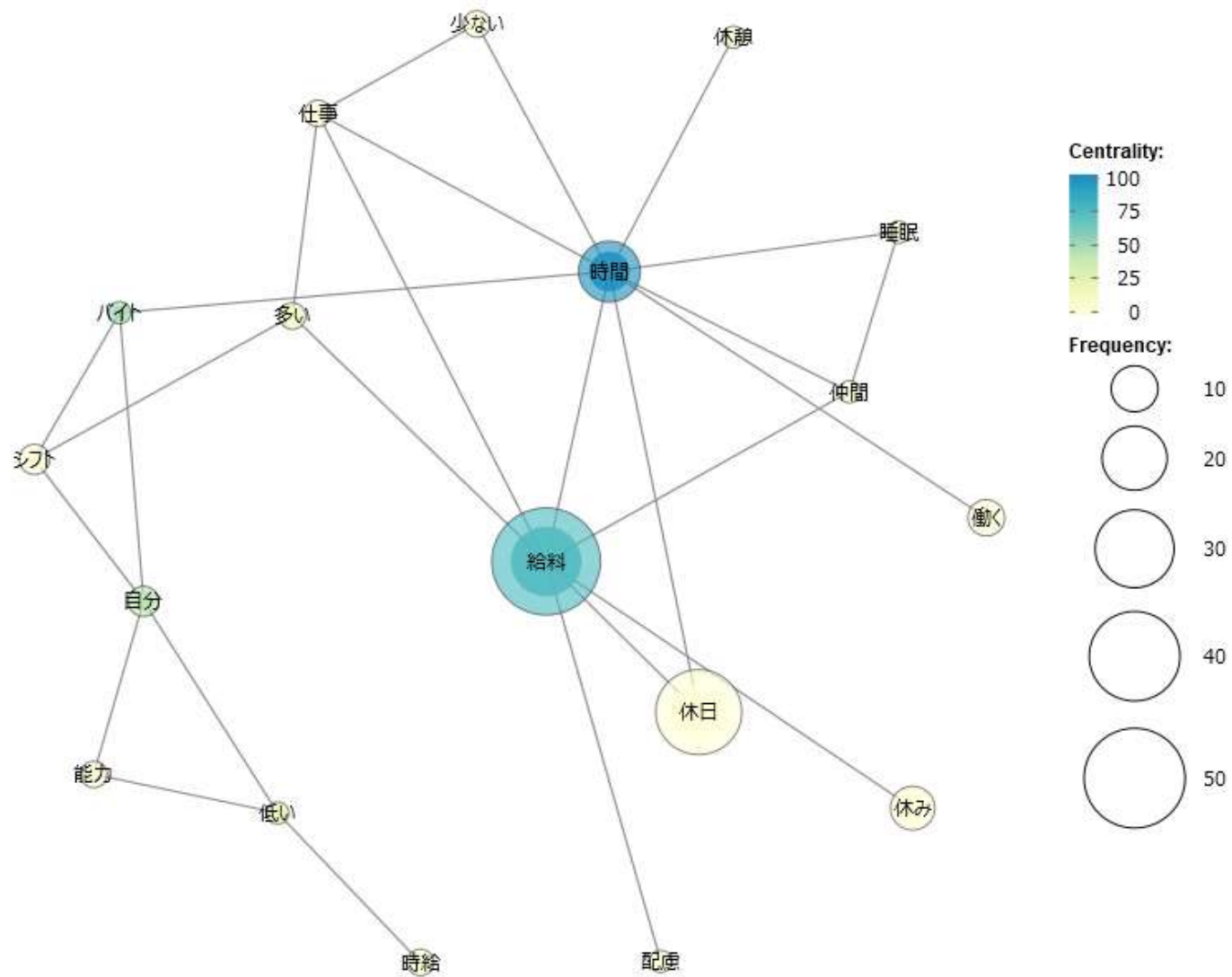
Q8中心性(媒介)
