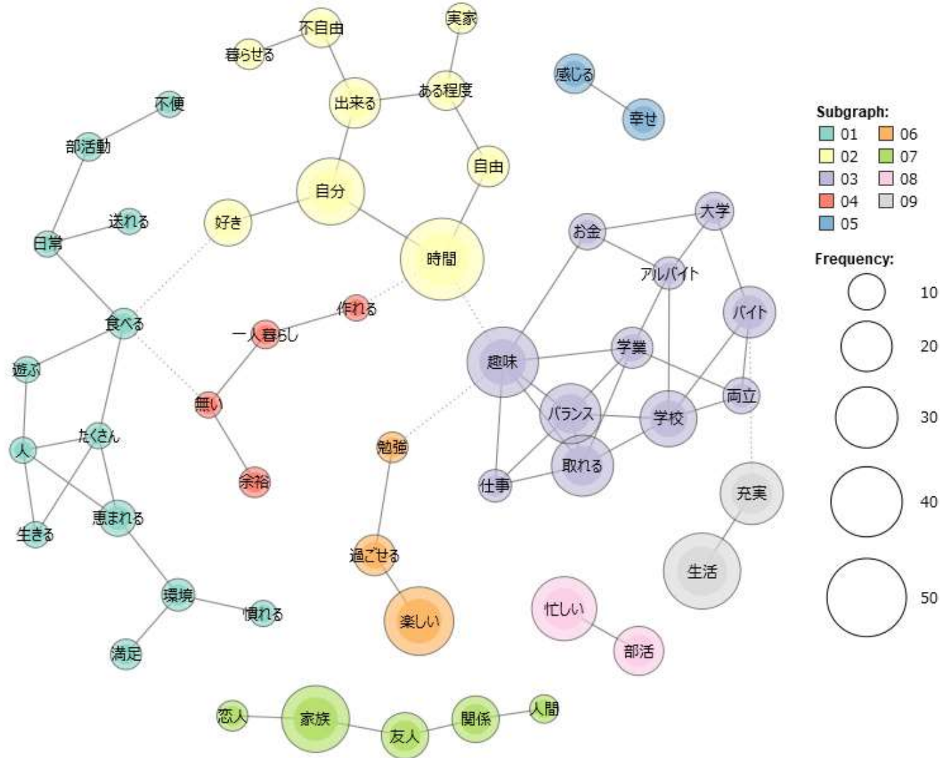
Q5サブグラフ(モジュラリティ)
