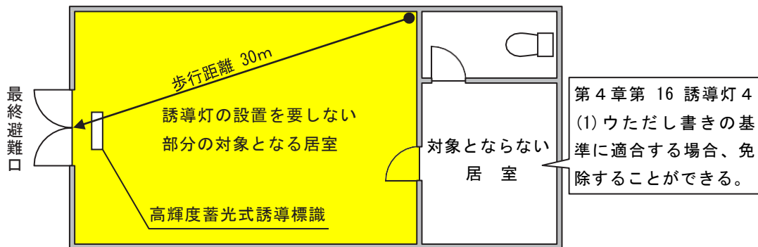
(地階に存する居室における誘導灯の設置免除の対象となる例)
