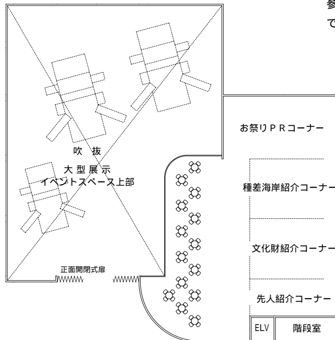
2 階平面図
