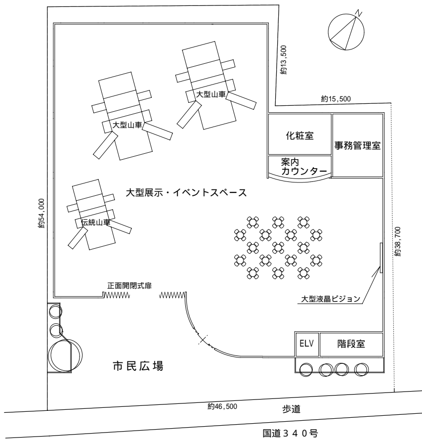
1 階平面図
